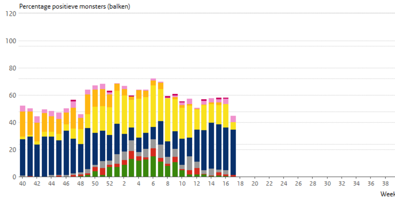
Luchtwegvirussen in monsters van deelnemers met zelfgerapporteerde acute luchtwegklachten Per week
